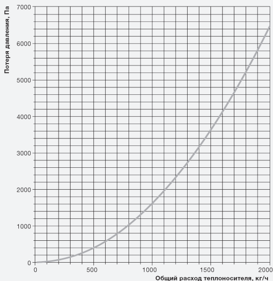
Потери давления в паре коллекторов
