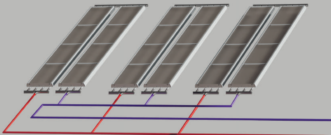
Схема Тихельмана
