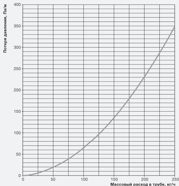
Потери давления в паре коллекторов
