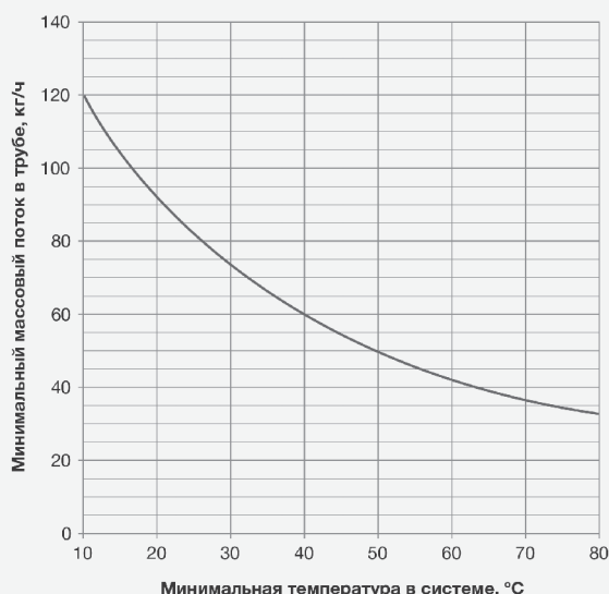
Минимальный массовый поток
